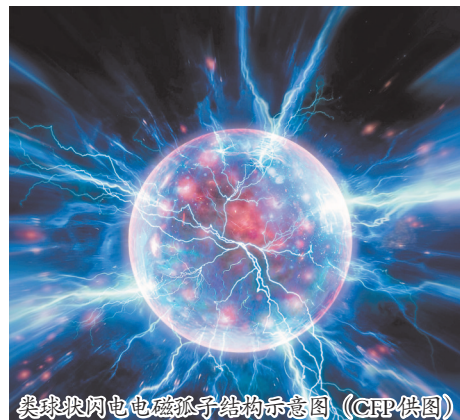
球状闪电电磁孤子结构示意图(CRP供图)
